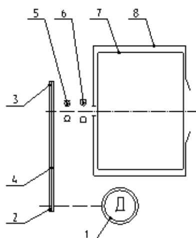
Кинематическая схема машины
